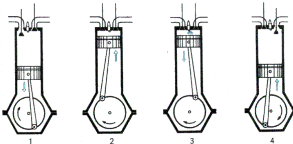
Znázornění pracovního cyklu čtyřdobého zážehového motoru
